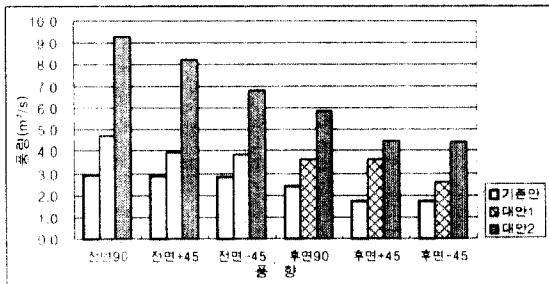
그림10. 유입풍량의 비교(Unit 7)
